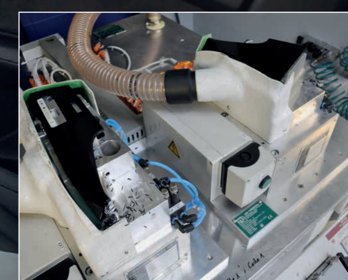
Die Vorrichtungen sind auf zwei Bauteile je Platte ausgelegt, die gleichzeitig bearbeitet werden.
