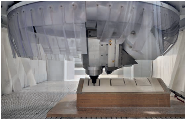
▲ Bearbeitung der Außenblende eines Gewürzregals aus Acrylglas.
