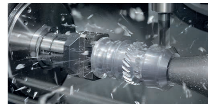
Drehfunktion der Rundachse: Werkstücke können vollständig gedreht und in einer Aufspannung bearbeitet werden.
